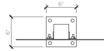
TOP VIEW SCALE: N.T.S.
